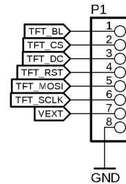
TFT Header
